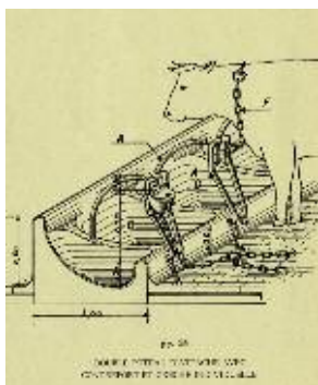
Systeem voor het vastbinden van runderen in een stal, midden van de 20ste eeuw (overgenomen uit: Les étables modernes , Ministerie van Landbouw en Bevoorrading, Algemene Directie Land- en Tuinbouw, Dienst Rurale Technieken, 1942, fig. 22).
