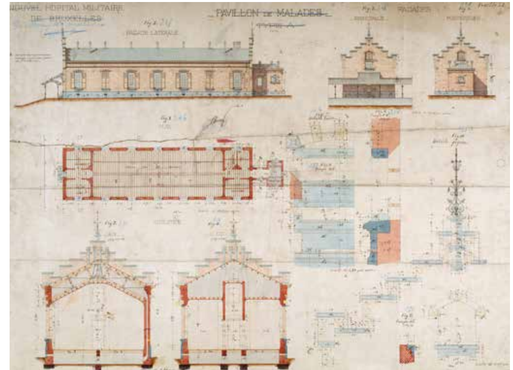
Plan van een ziekenpaviljoen in het militair hospitaal van Elsenne, 1884.
