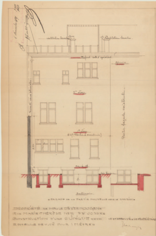
Afb. 3b Gevel op de lichtput met het glazen dak dat de operatiezaal verlicht (Archief Sint-Joost-ten-Node, PU 7483).
