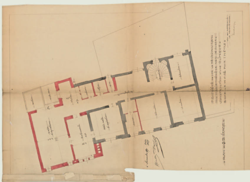
Afb. 3a Gebouw in Maria-Theresiastraat 102-104. Plan van de verdieping van de operatiezaal (Archief Sint-Joost-ten-Node, PU 7483, in 1907).
